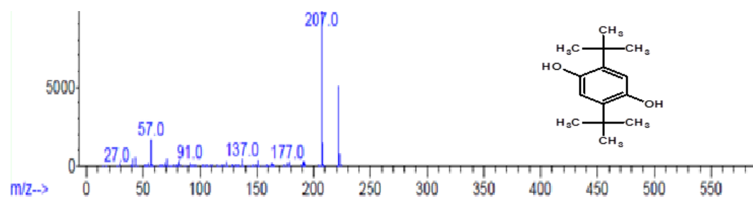
Fig. 1.12: 1,4-Benzenediol, 2,5-bis(1,1-dimethylethyl)-
