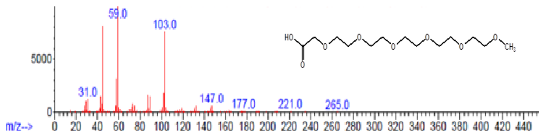
Fig. 2.1: 2-(2-(2-(2-(2-methoxyethoxy)ethoxy)ethoxy)ethoxy)ethoxy) acetic acid
