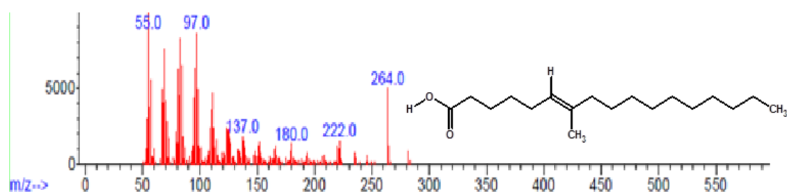
Fig. 1.15: 6-Octadecenoic acid
