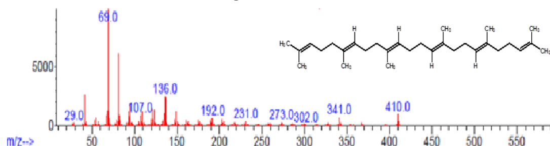
Fig. 1.16: Suprane
