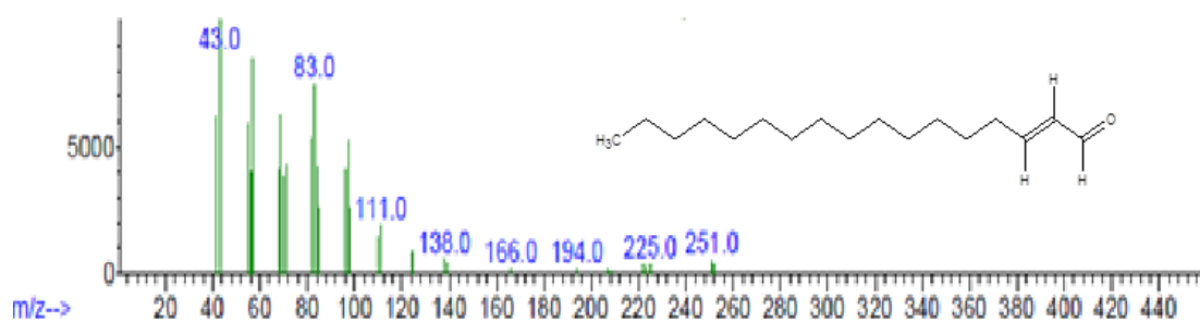
Fig. 1.2: 2-Heptadecenal
