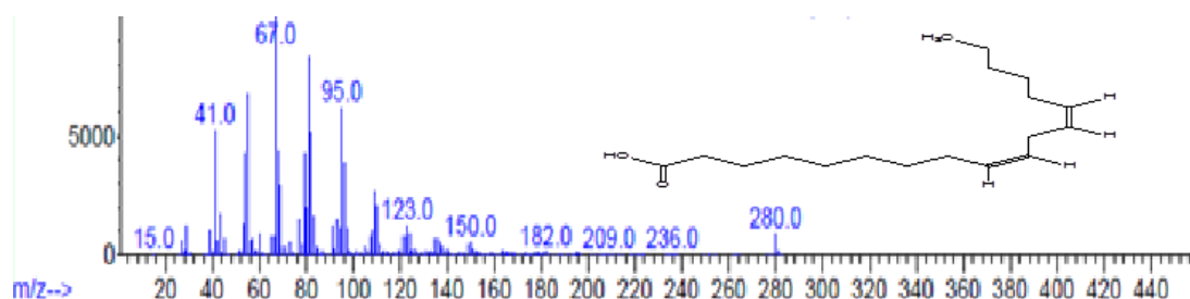
Fig. 1.3: 9, 12-Octadecadienoic acid (Z,Z)-
